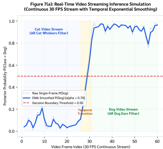
รูปที่ 7: การจำลองระบบสตรีมมิงวิดีโอแบบเรียลไทม์: (a) เส้นเวลาความน่าจะเป็นและการสลับโหมดฟิลเตอร์ (b) การจำลองระบบแปะฟิลเตอร์ AR หูแมว/หูหมี เทียบกับ หูสุนัข/จิ้งจอก บนใบหน้า
